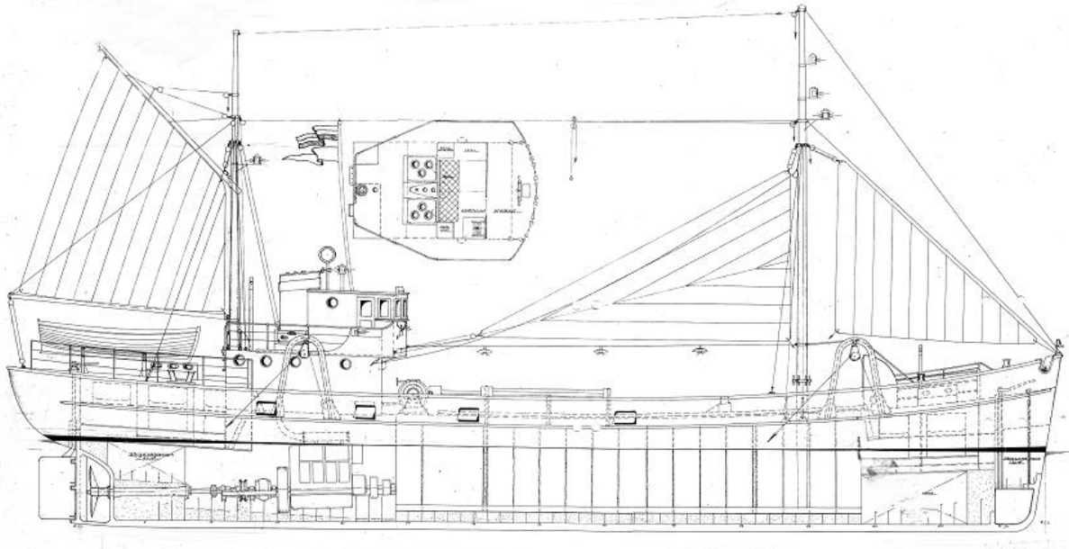
Zijaanzicht Noordster met tuigplan
